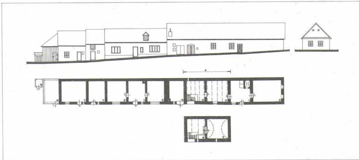
Pri vinohradoch č. 58. Spoločný dvor zložený z dvoch bytových jednotiek. Predná predstavuje tradičný vinohradnícky dom s dvoma obytými miestnosťami. Atypická je prístavená komora so samostatným vstupom. 1 – kuchyňa, 2 – izba, 3 – prešovňa, 4 – podpivničená časť, 5 – pivnica, 6 – komora, 7 – maštal, 8 – kôlna, 9 – chliev
