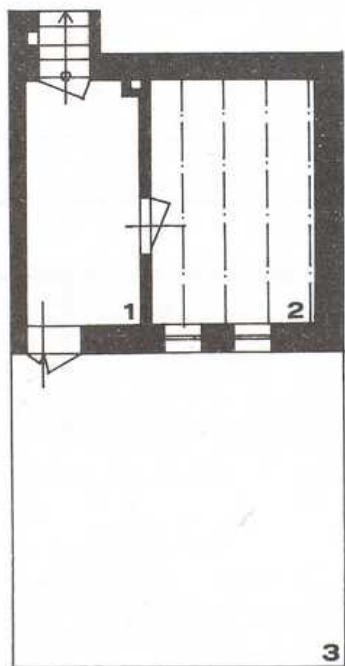
Zvončeková č. 19. Obydlie bezzemka zo začiatku 20. storočia. 1 – kuchyňa, 2 – izba, 3 – záhrada Pri vinohradoch č. 49 – dom I. 1 – maštal, 2 – komora, 3 – kuchyňa, 4 – izba; Situácia – domy 1, 2, 3, 4, 5 – dreváreň, chliev, 6 – kôlna
